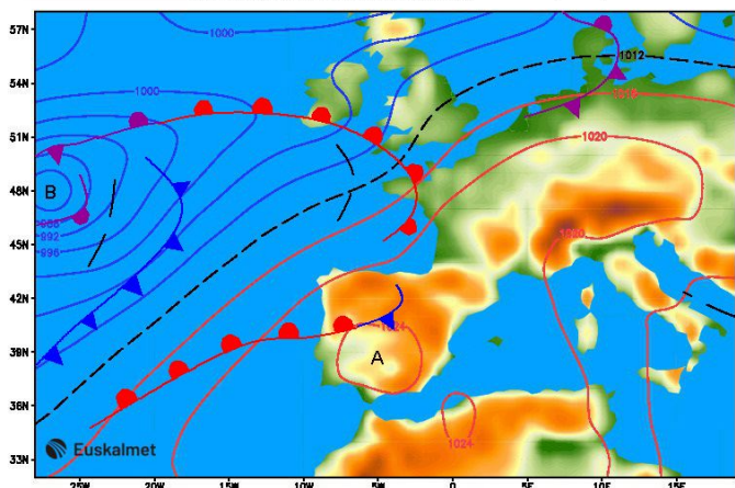
Fronteak eta Presioa itsas mailan (mb) 2024/02/13 12:00 Frentes y Presión nivel mar (mb)
