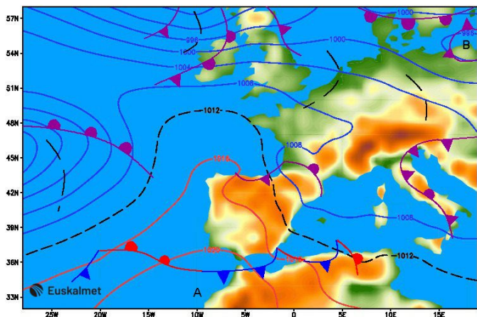
Fronteak eta Presioa itsas mailan (mb) 2024/02/12 12:00 Frentes y Presión nivel mar (mb)
