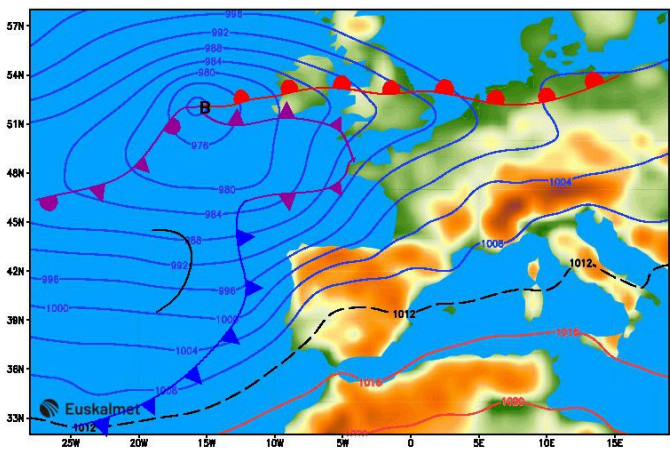
Fronteak eta Presioa itsas mailan (mb) 2024/02/08 12:00 Frentes y Presión nivel mar (mb)
