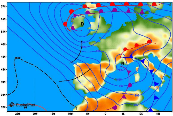
Fronteak eta Presioa itsas mailan (mb) 2024/02/10 12:00 Frentes y Presión nivel mar (mb)
