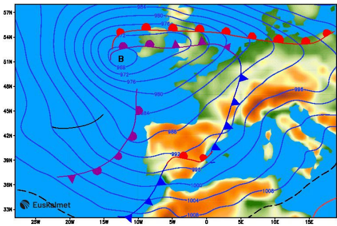
Fronteak eta Presioa itsas mailan (mb) 2024/02/09 12:00 Frentes y Presión nivel mar (mb)
